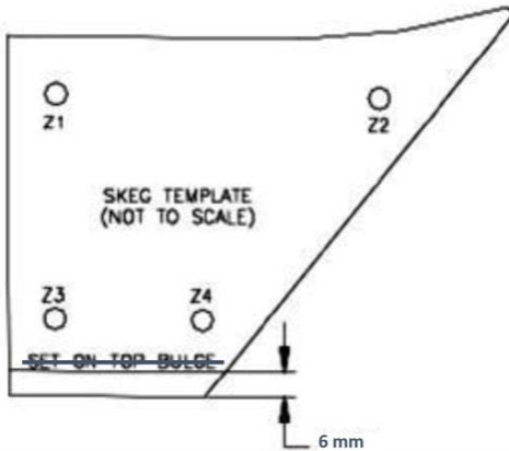
↑ Skeg Template
